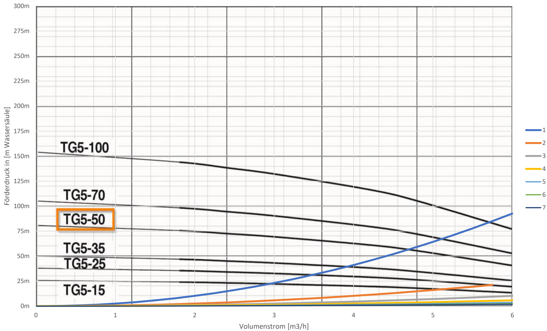
Pumpenkennlinie mit Anlagenkennlinien in Abhängigkeit der Anzahl Kreise
